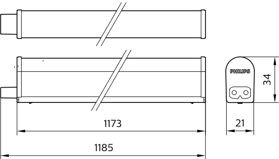
BN068C LED12/NW L1200 TH G2
